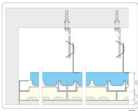
Estructura de perfil colgante de encaje
