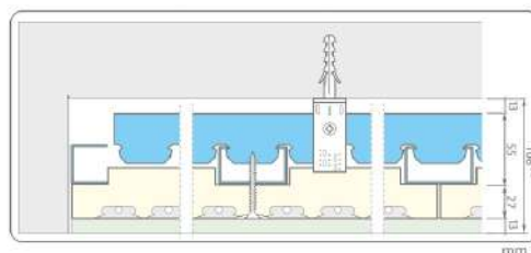
Estructura con perfil de encaje
